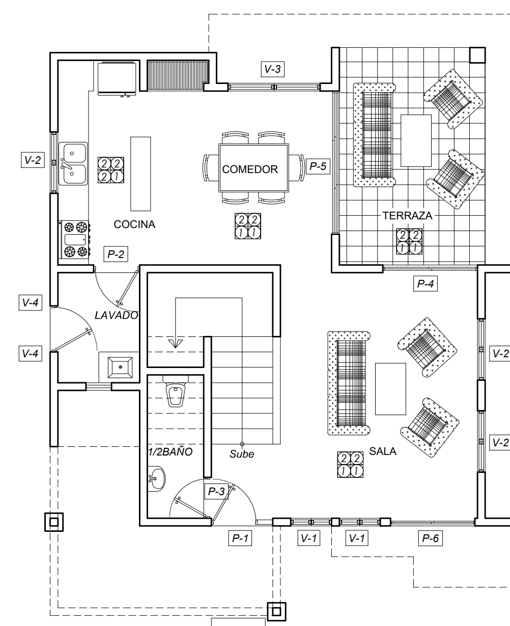
PLANTA ARQUITECTONICA AMUEBLADA ESC. 1:75 1ER. NIVEL
