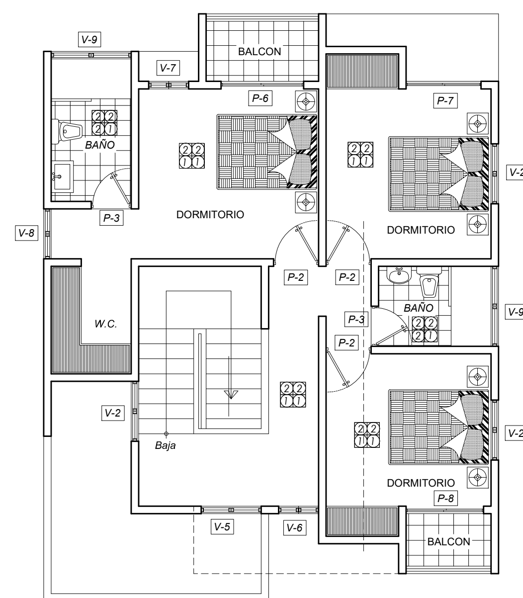
PLANTA ARQUITECTONICA AMUEBLADA ESC. 1:75 2DO. NIVEL
